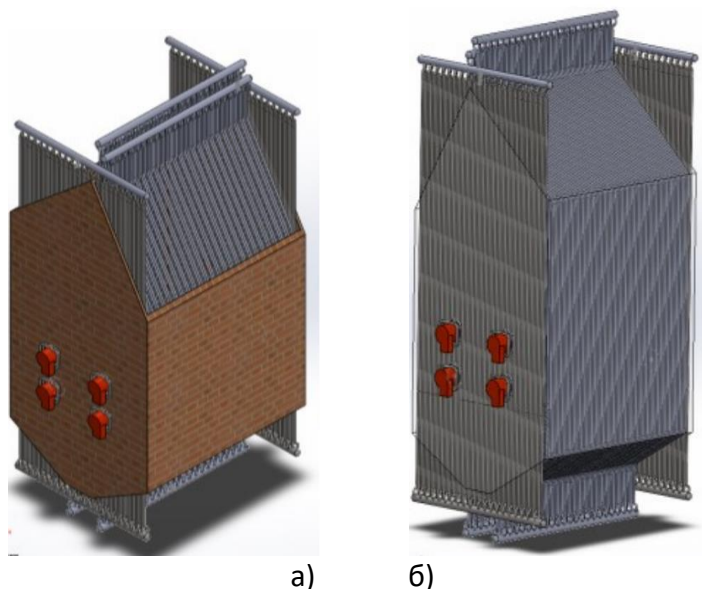
Рис.1 Зовнішній вигляд моделі котла ГМ-50 (а), та модель котла без обмуровки (б)
