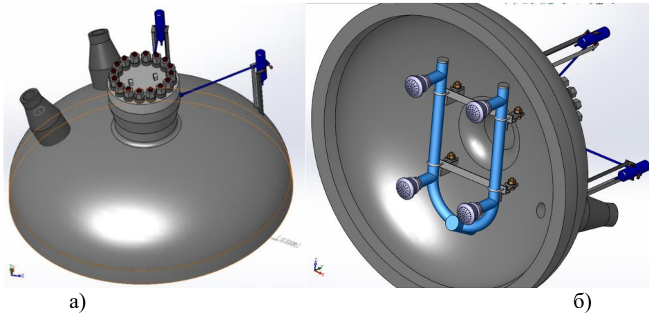
Рисунок 2.4 - Вид зверху (а), вид знизу (б) кришки компенсатора тиску
