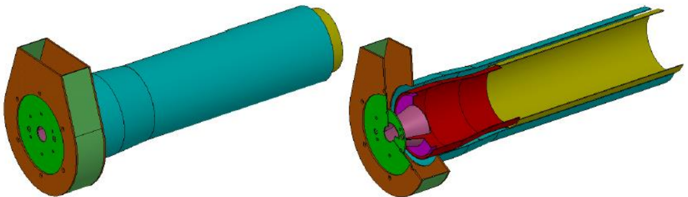
Рисунок 2.2 – Моделі пальника ДВС.
