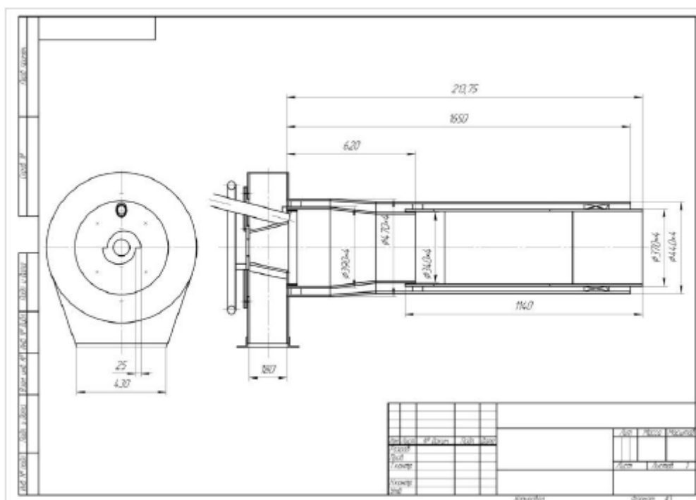
Рисунок 2.1 – Кресленник пальника ДВБ
