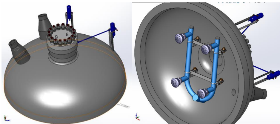
Рисунок 2.4 - Вид зверху (а), вид знизу (б) кришки компенсатора тиску
