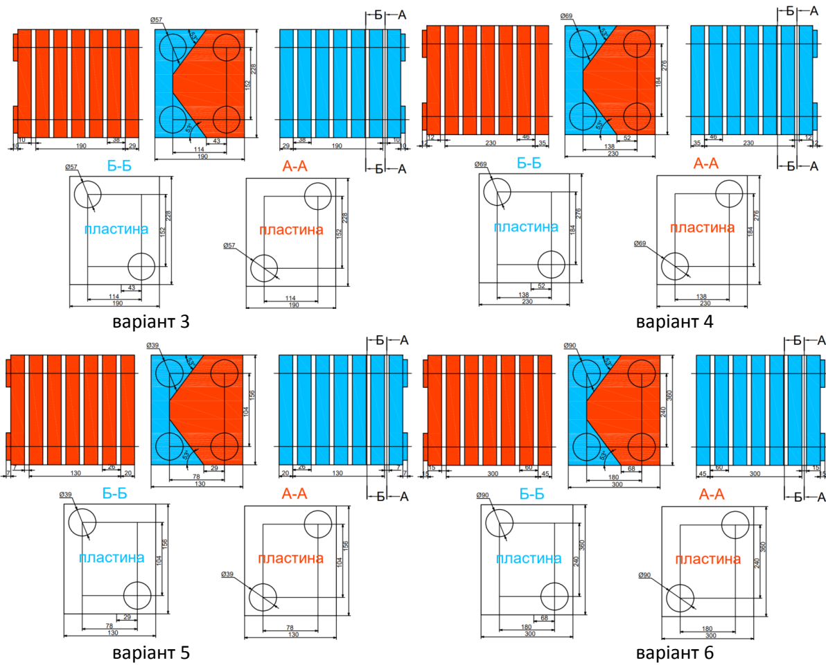
Рис. 1 – Теплообмінні апарати
